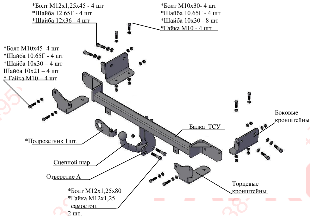
Рис.1 Тягово-сцепное устройство 7330.
